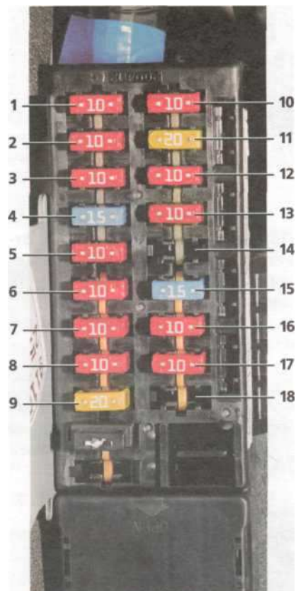
Монтажный блок предохранителей в салоне: 1 — предохранитель 10 А цепи указателей поворота; 2 — предохранитель 10 А цепей ABS, контрольных ламп в комбинации приборов; 3 — предохранитель 10 А цепи комбинации приборов; 4 — предохранитель 15 А цепи подушки безопасности; 5 — предохранитель 10 А цепей блока управления двигателем, ламп света заднего хода, блока управления автоматической коробкой передач; 6 — предохранитель 10 А цепи электрического привода блокировки двери; 7 — предохранитель 10 А цепи аварийной сигнализации; 8 — предохранитель 10 А цепи сигналов торможения; 9 — предохранитель 20 А цепи обогрева заднего стекла; 10 — предохранитель 10 А цепей обмоток реле блок-фар, электростеклоподъемников, омывателя блок-фар, вентилятора теплообменника конденсатора системы кондиционирования, вентилятора радиатора системы охлаждения двигателя, противотуманных фар, противотуманного света в задних фонарях; 11 — предохранитель 20 А цепи очистителя и омывателя ветрового стекла; 12 — предохранитель 10 А цепи обогрева сиденья (опция); 13 — предохранитель 10 А цепи ABS; 14 — резервное гнездо предохранителя; 15 — предохранитель 15 А цепи прикуривателя; 16 — предохранитель 10 А цепи наружных зеркал с электроприводом; 17 — предохранитель 10 А цепи кондиционера; 18 — резервное гнездо предохранителя
