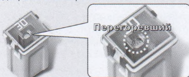
Предохранитель патронного типа
