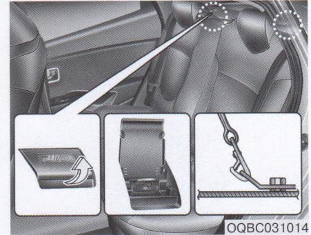
Крепление детского кресла с помощью системы привязных креплений "Tether Anchor" (при наличии)
